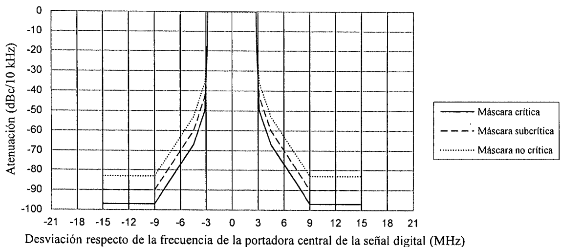
Cuadro N° 3 Especificación de la máscara de transmisión digital
